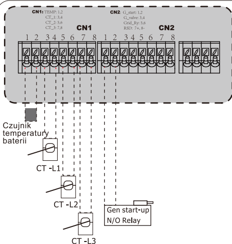
Falownik
